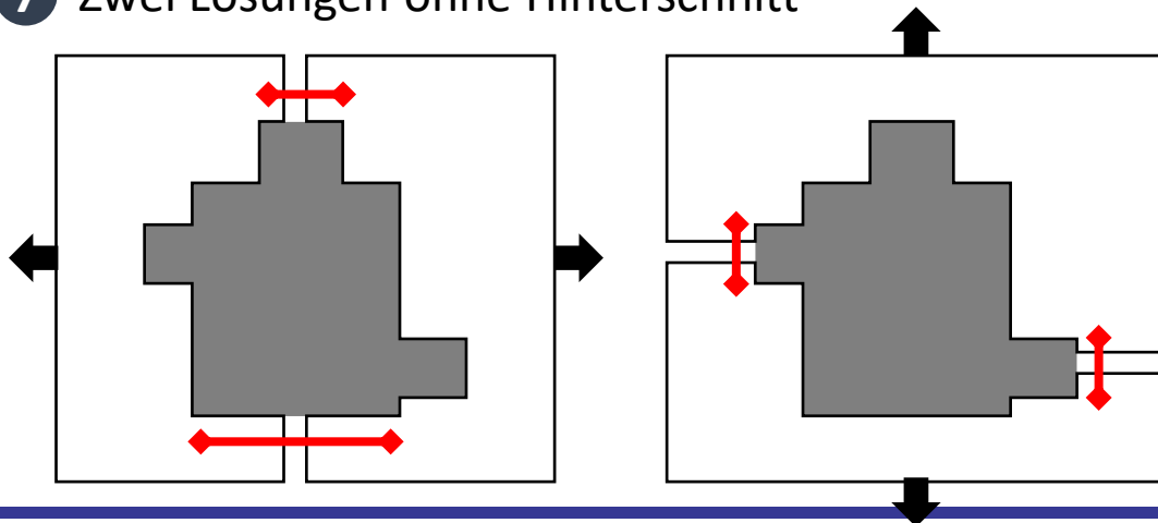
7 Zwei Lösungen ohne Hinterschnitt
