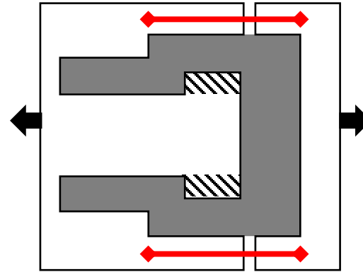
2 Einzige Lösung, Hinterschnitt unvermeidbar
