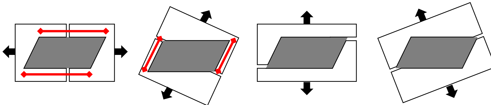
3 Mehrere Lösungen möglich ohne Hinterschneidungen
