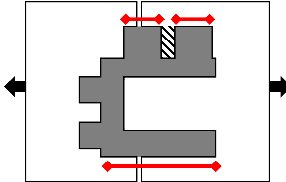
6 Einzige Lösung mit kleinstem Hinterschnitt
